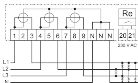
Jednosadzbový elektromer s relé
